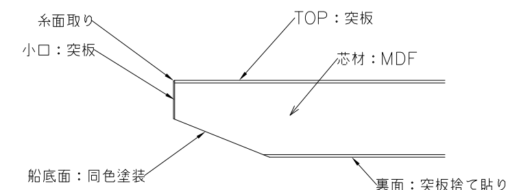
【天板小口詳細図 S=1：2】
